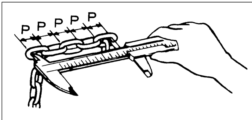
Joonis 5 Keti mõõtmete kontrollimine
