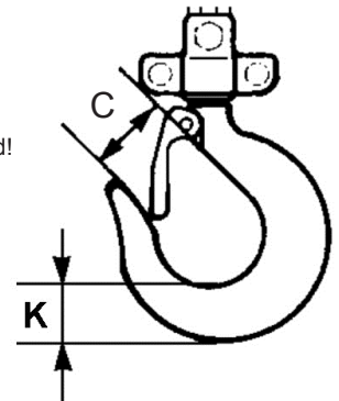
Fig. 4 Lasthaak
