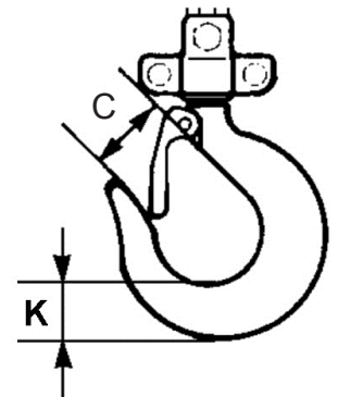
Joonis 4 Tõstekonks
