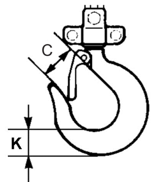
Imag. 4: Gancho de carga
